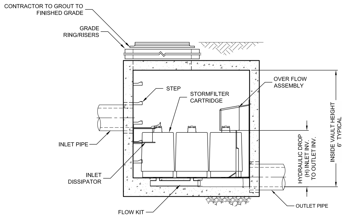
SECTION A-A
