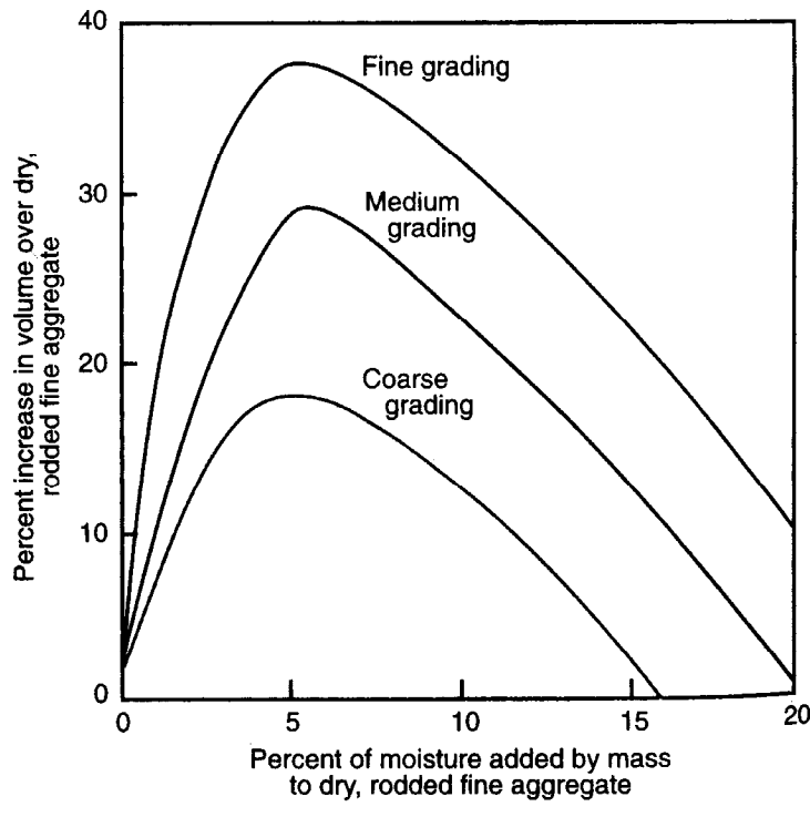
Fig. 1-Sand bulking (Kosmatka et al. 2002) .
