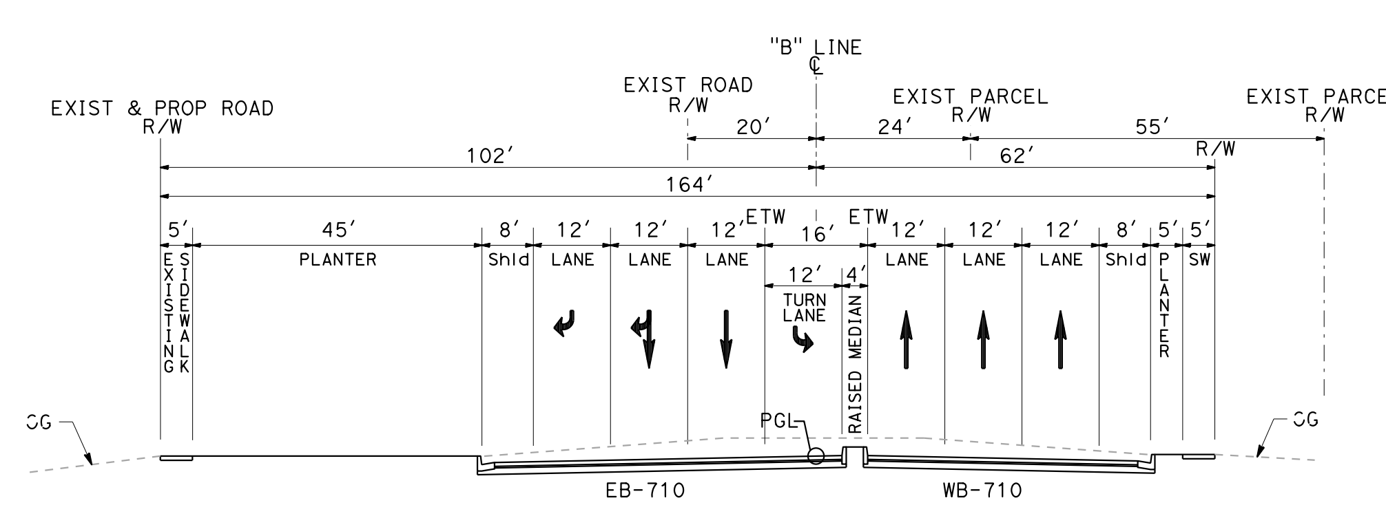
SECTION A-A SR-710/MONTERREY RD NTS
