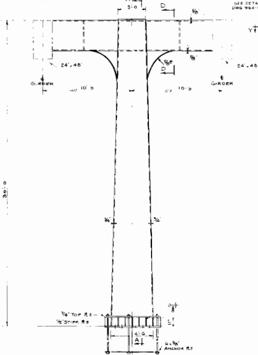
ELEVATION
