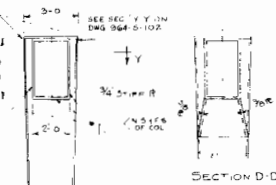
SECTION D-D
